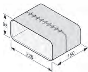
Forlængerstykke DFK-L
